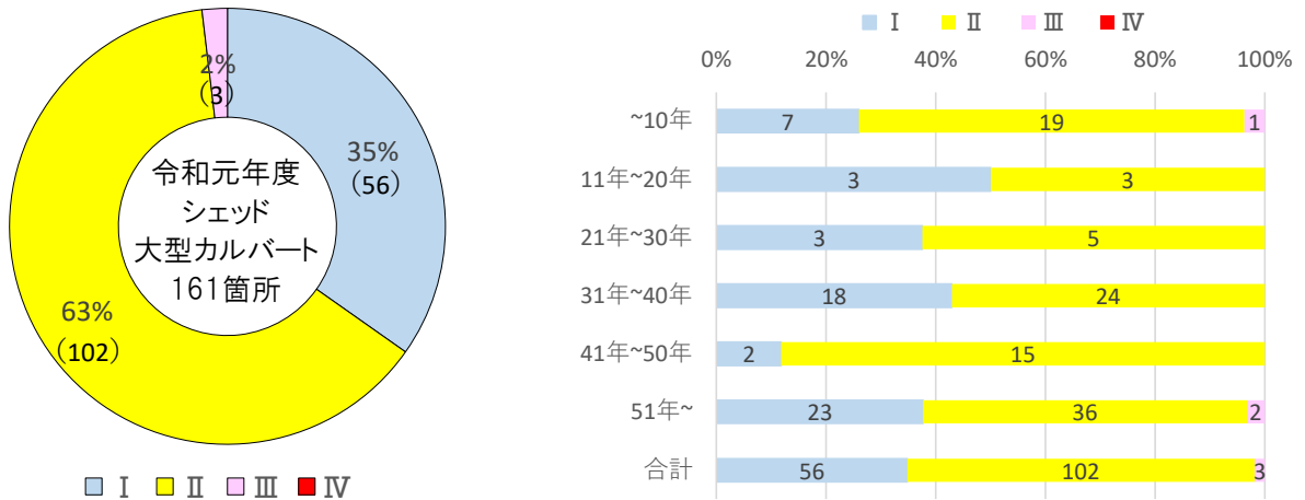
○判定区分と建設経過年度 (シェッド、大型カルバート)
