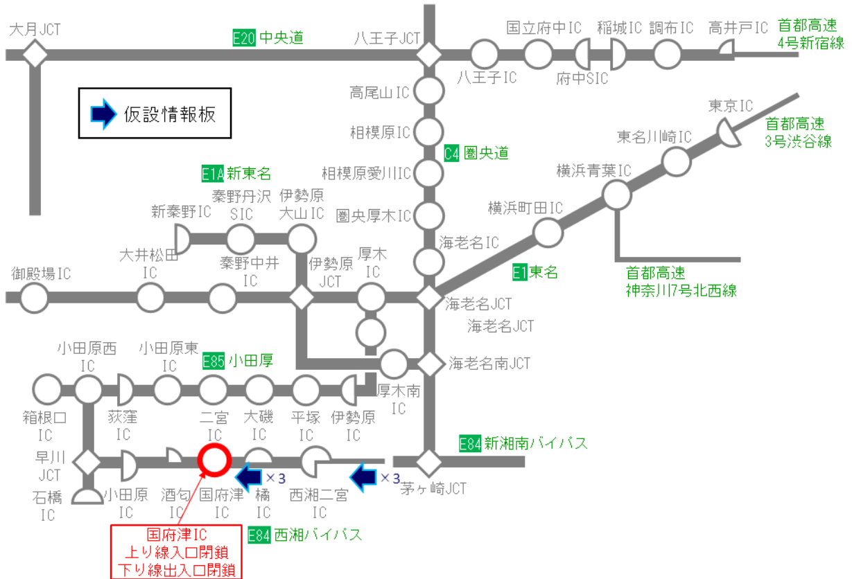
【夜間 IC 閉鎖(出口閉鎖)箇所手前への仮設情報板の設置予定箇所】
