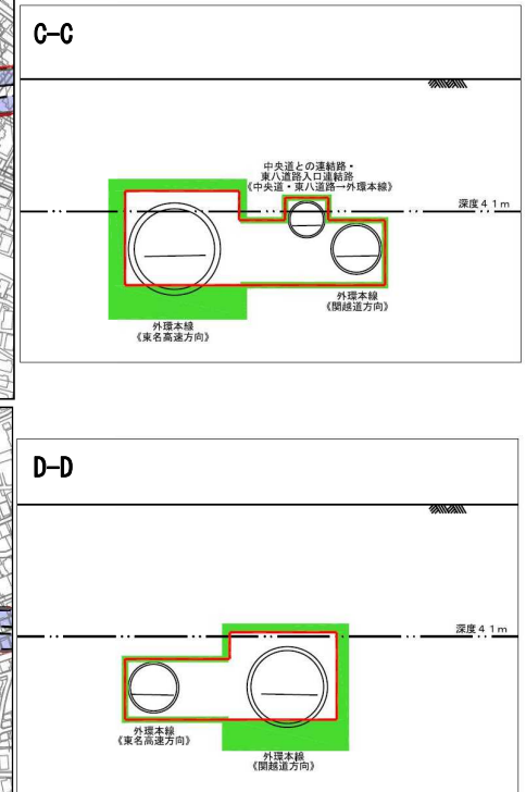
【断面図】
