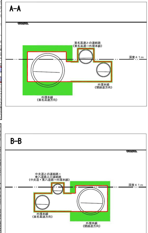
【断面図】
