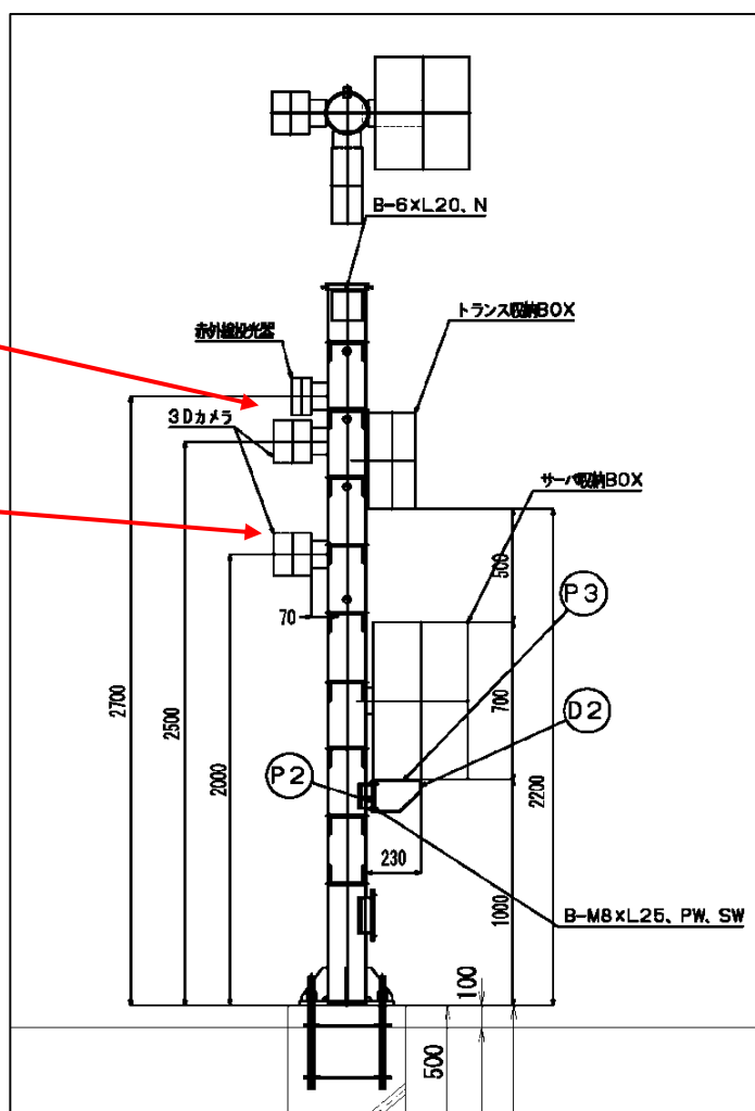
設置図面
