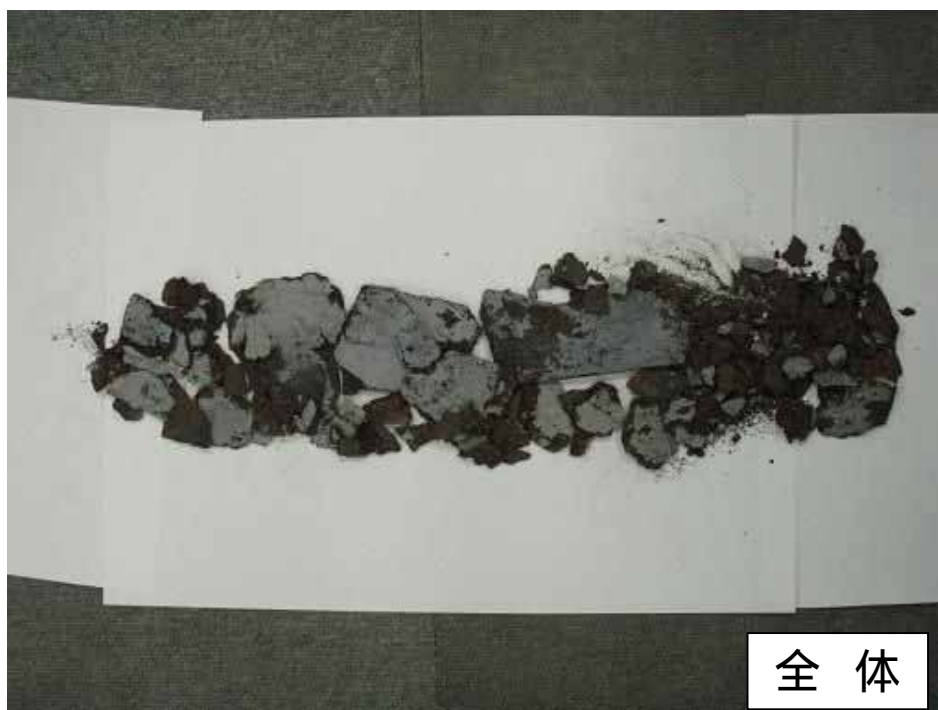
調布高架橋ジョイント部から落下した錆片
