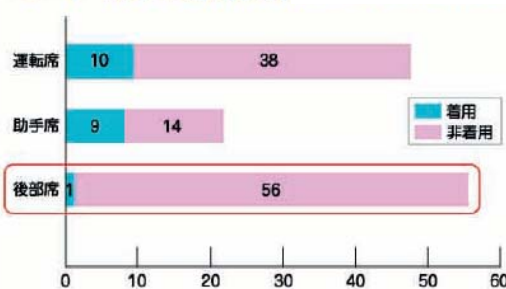
●車外放出事故死傷者数と乗車位置・シートベルトの着用状況 (警察庁道路局調べ) H17年、高速道路
