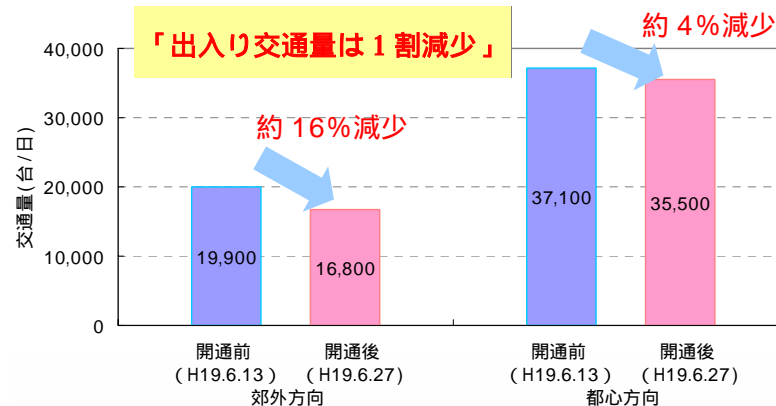
中央道八王子ICの出入り交通量
