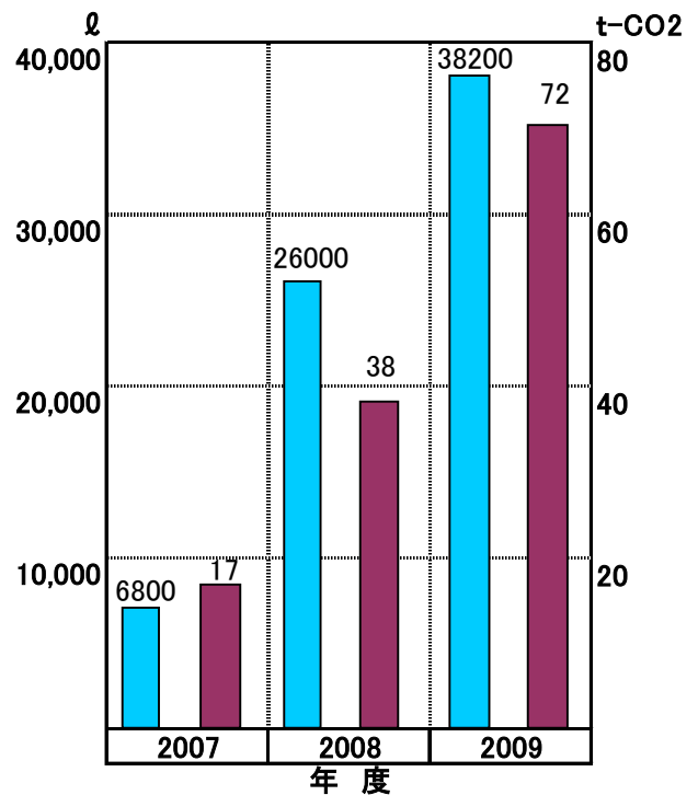
燃料使用量とCO2抑制量
