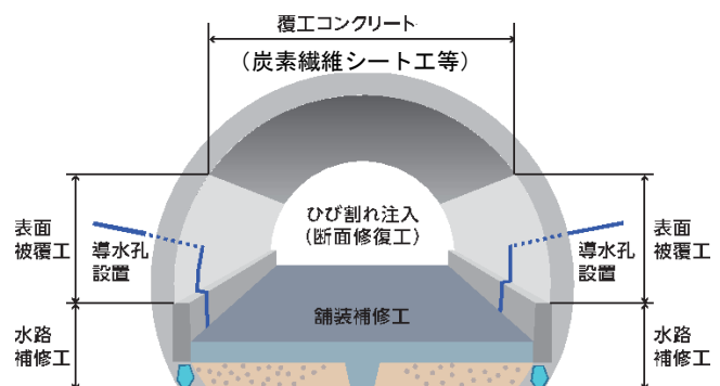
トンネルの補強工事
