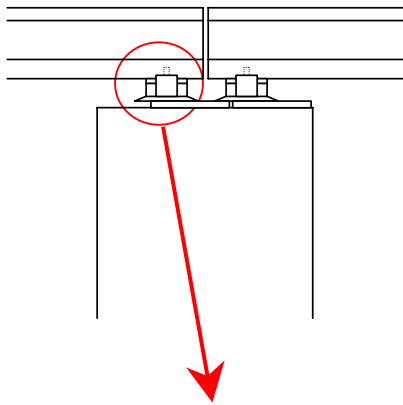
橋梁支承部縦断面図 (橋梁側面)
