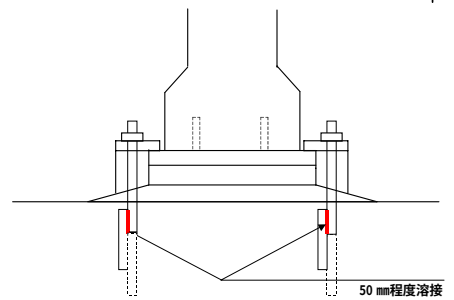
支承部詳細図 (溶接処理の事例)
