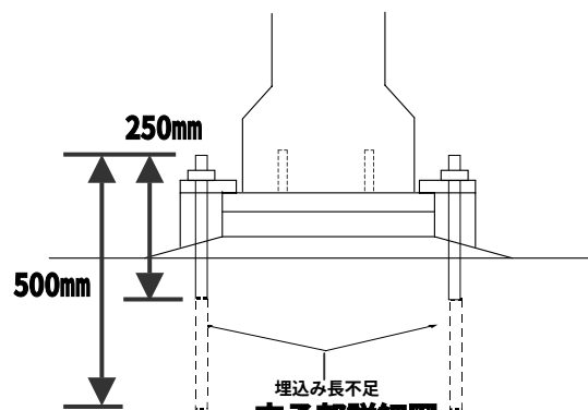
支承部詳細図 (埋込み長不足の事例)
