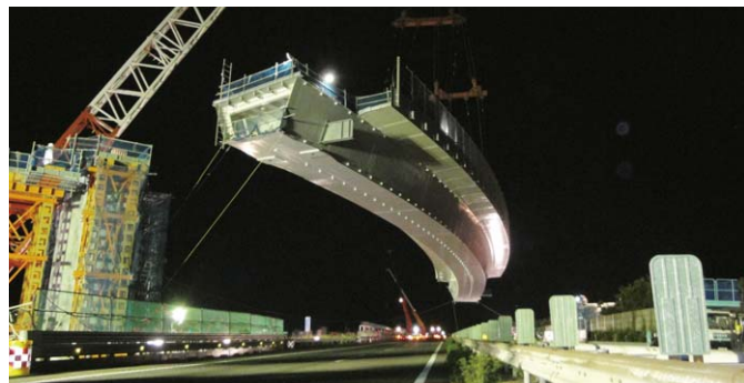
夜間通行止め架設のイメージ(2011.9.6 名神高速道路 養老ジャンクション)
