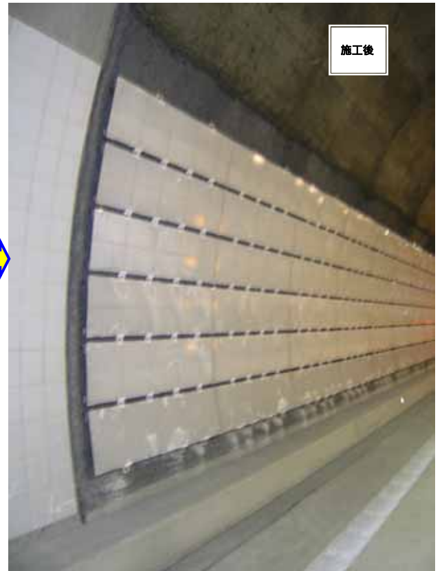
( 飛驒トンネルのタイルパネル補強対策写真 )
