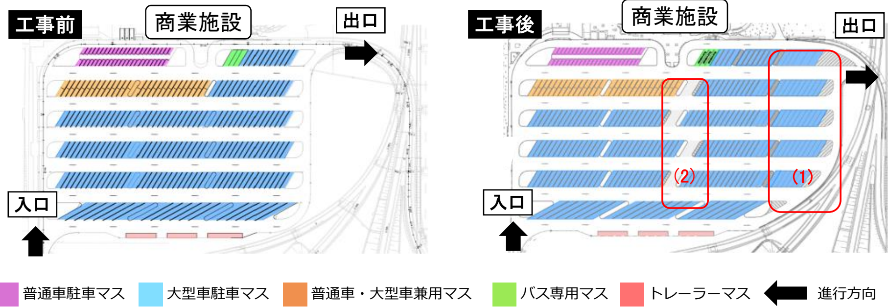
図-1 工事前後の駐車マス配置
