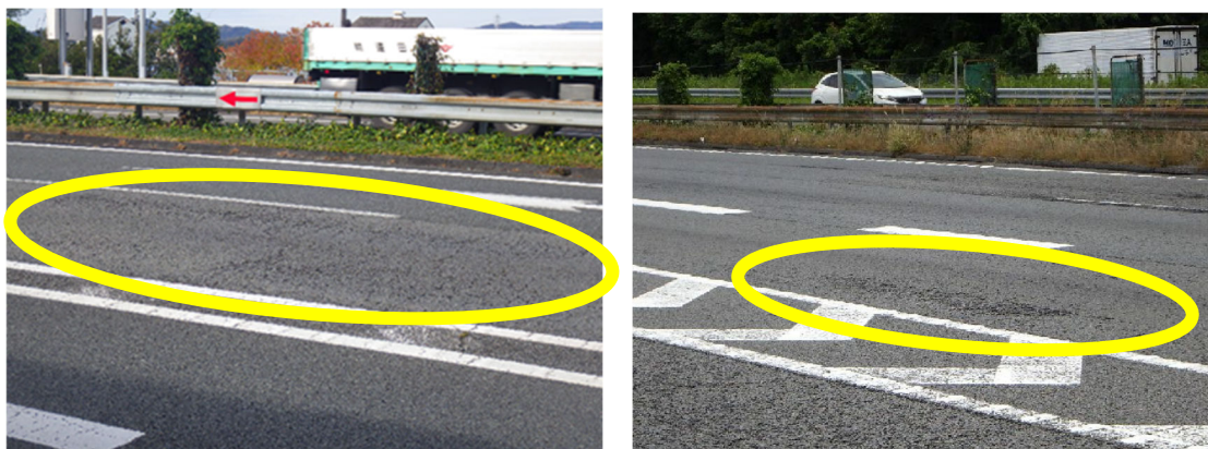
牧之原 SA(下り)入口付近の舗装損傷状況
