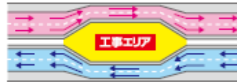
4車線を確保した車線シフト規制
