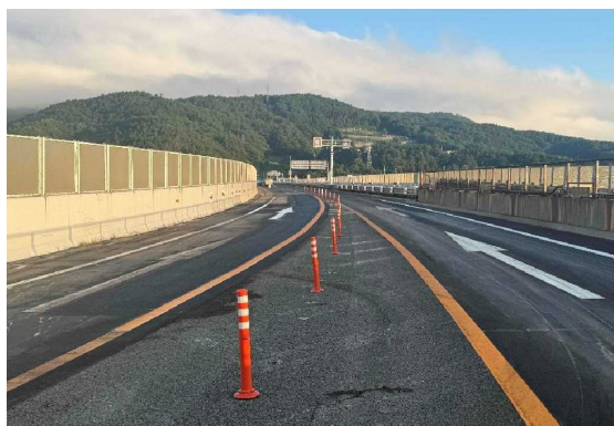
長野道(下り線)岡谷 JCT 車線分離標設置状況
