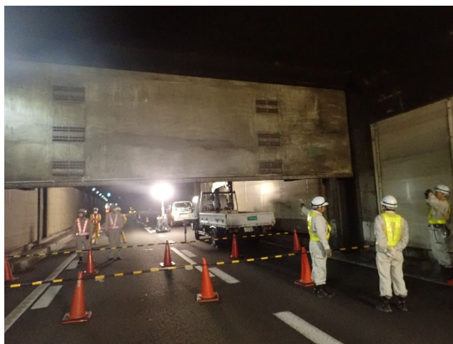
制水ゲートの点検
