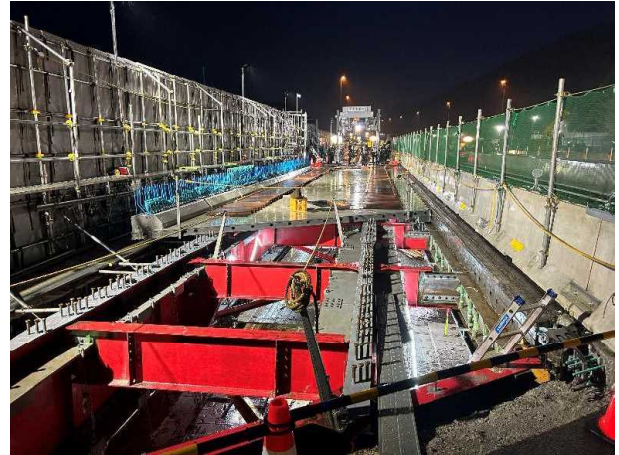
2024 年度名神集中工事 名神 河内橋での床版取替の状況写真
