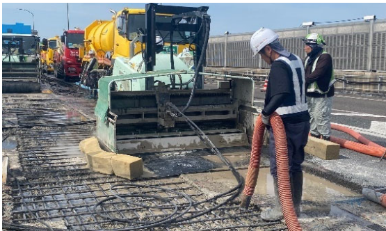
老朽化した床版の補修状況
