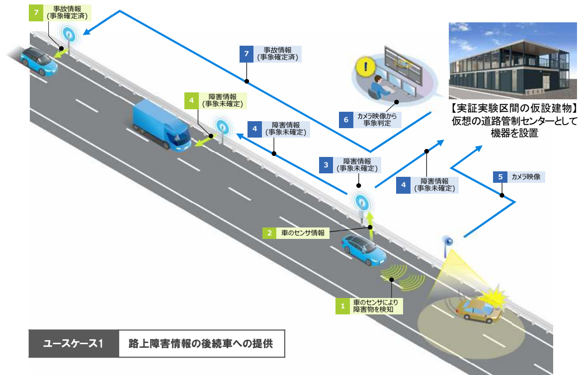
図1 路車協調実証実験で検証するユースケースの一例
