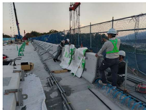
プレキャスト壁高欄の施工
