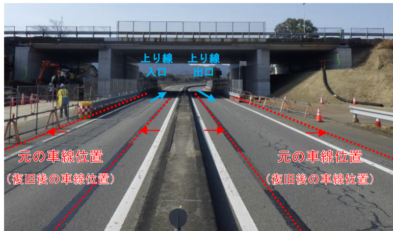
現況の車線シフト状況と復旧後の車線位置(イメージ)
