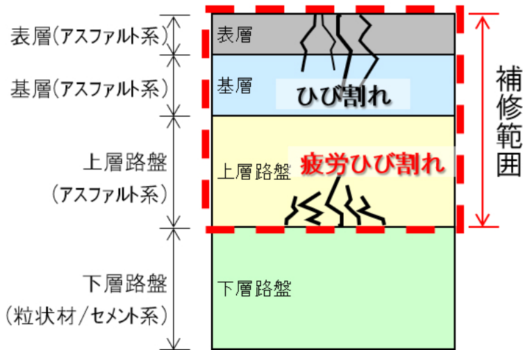
図-4 現在の打替え工法イメージ
