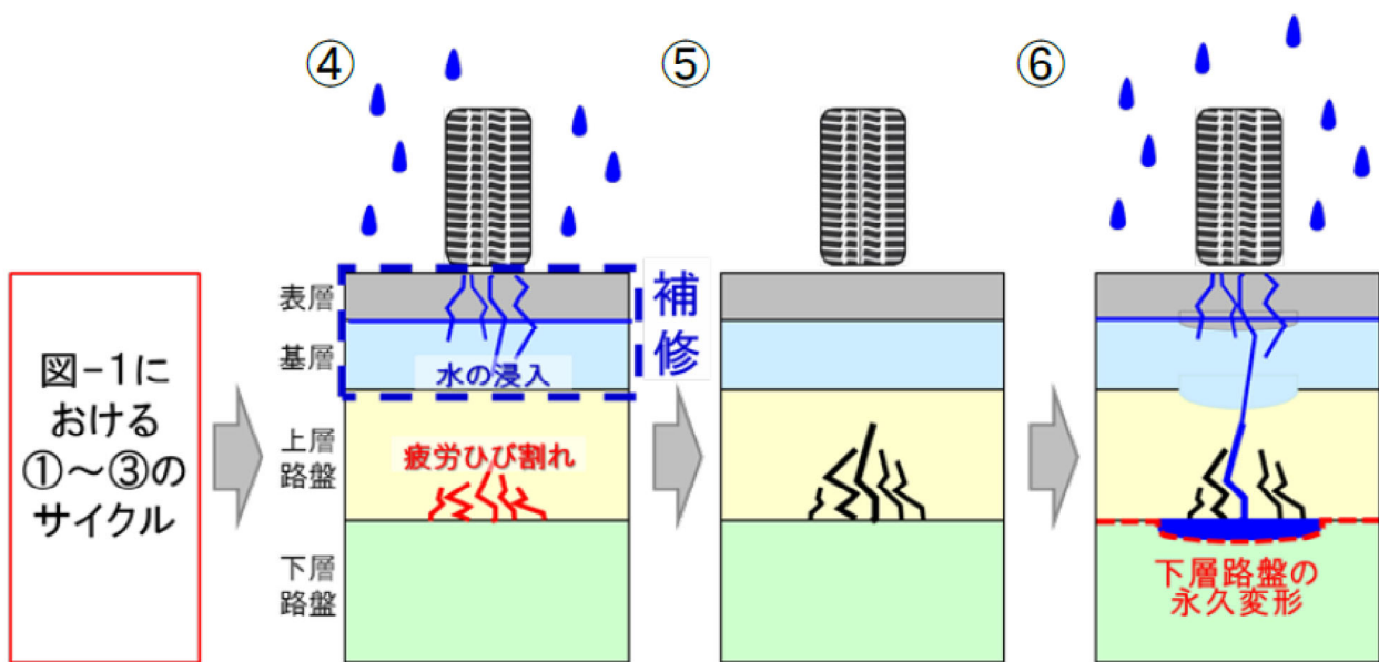
図-3 深層部における損傷メカニズム
