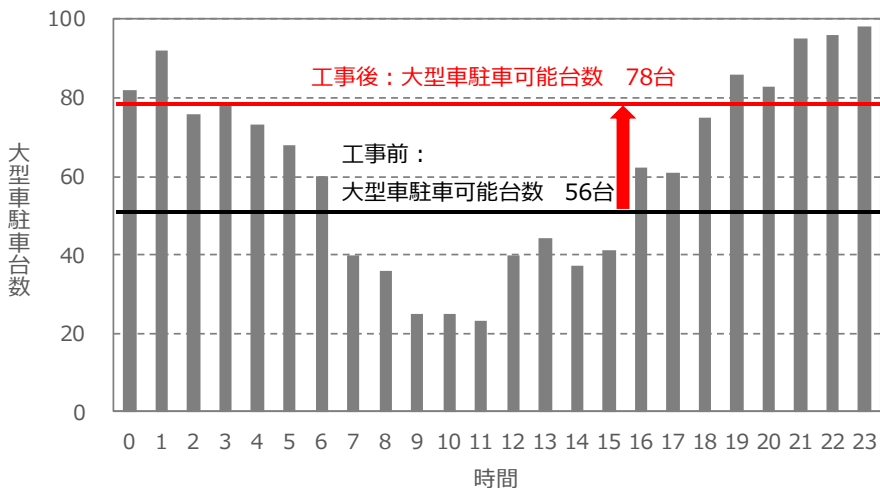
図 時間帯別大型車駐車状況(平日)と駐車可能台数(工事前後) 鈴鹿 PA(上り)
