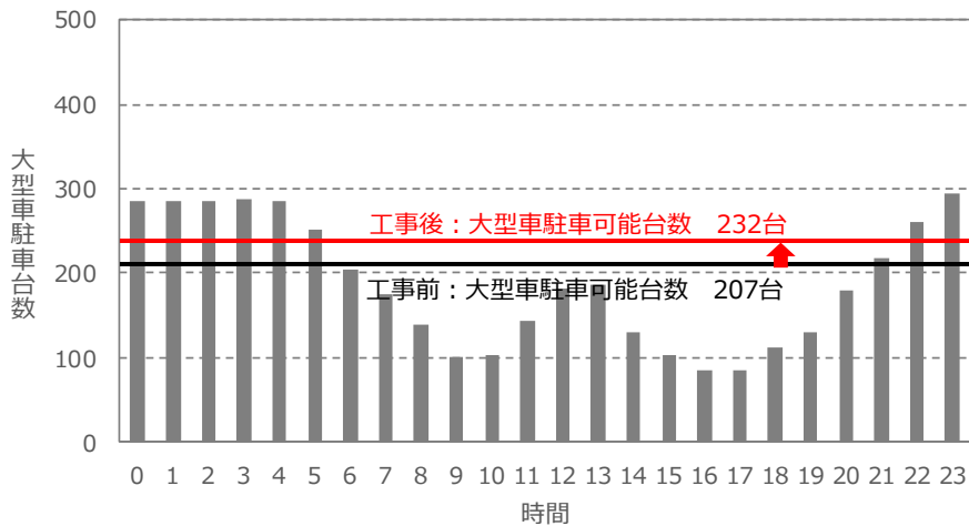
図 時間帯別大型車駐車状況(平日)と駐車可能台数(工事前後) 大山田 PA(下り)、御在所 SA(下り)、亀山 PA(下り)の合計
