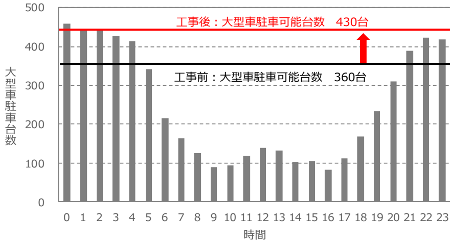
図 時間帯別大型車駐車状況(平日)と駐車可能台数(工事前後) 湾岸長島 PA(下り)、鈴鹿 PA(下り)、土山 SA(下り)の合計
