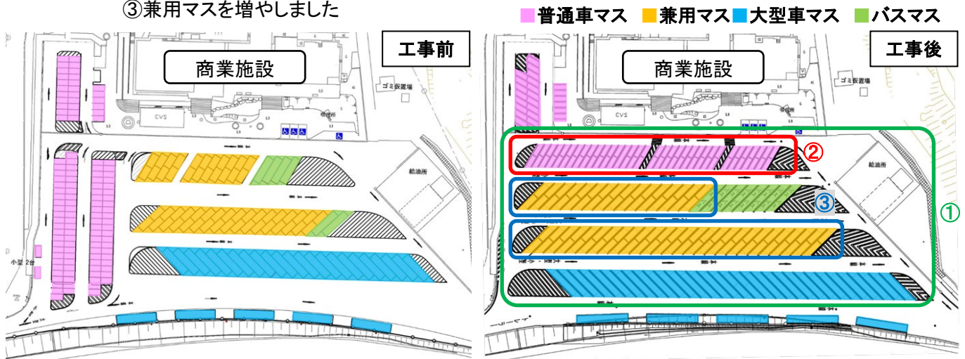
図2 駐車場レイアウトと変更点(左:変更前、右:変更後)
