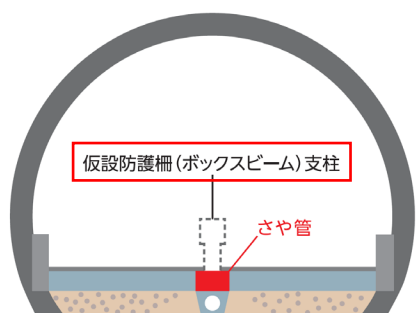
蒲原トンネル仮設防護柵位置
