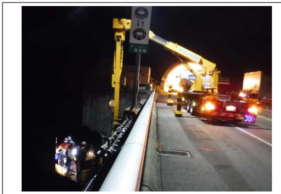
(橋梁点検車を用いた橋梁下面および橋桁の点検)
