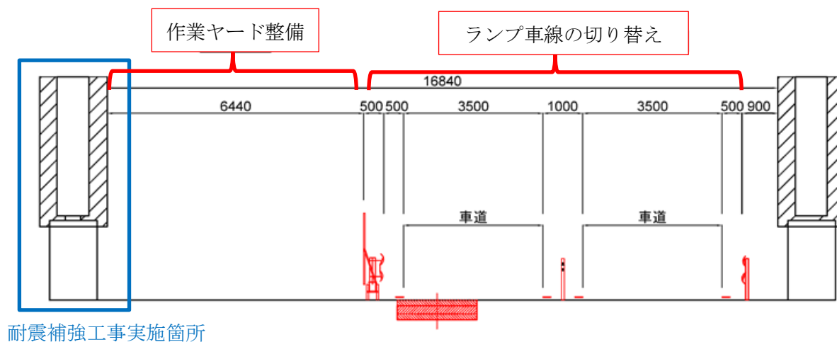
切り替え後断面図
