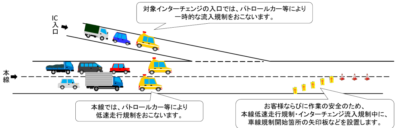
【低速走行規制及び流入規制の例】
