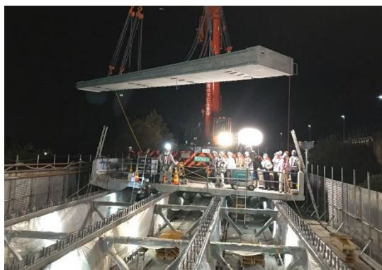
プレキャスト床版の施工状況
