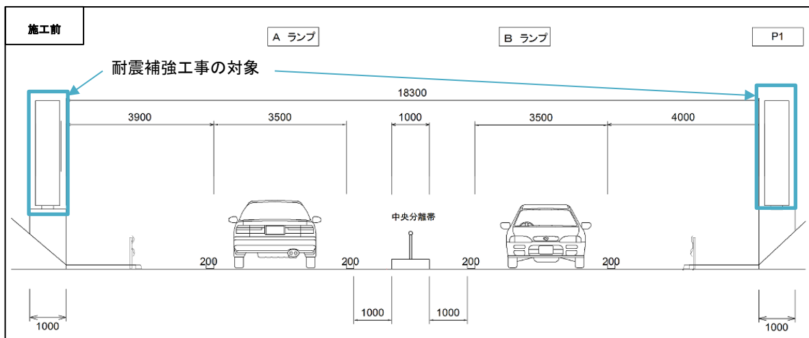
【ランプ断面図】
