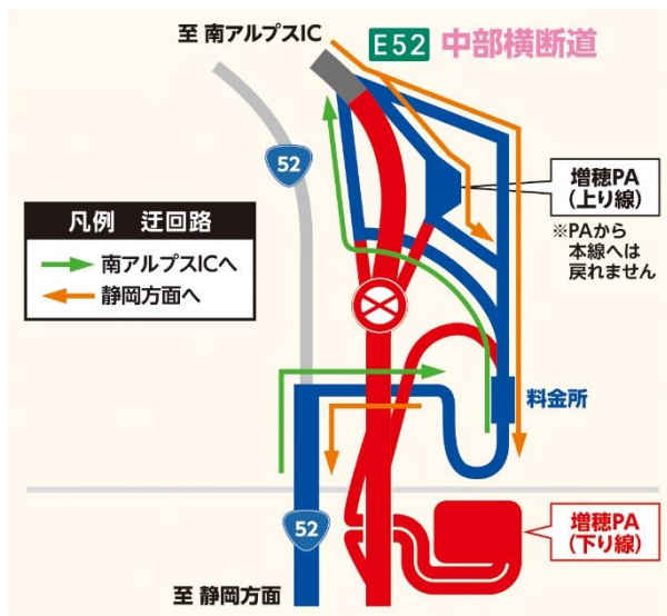
○増穂インターチェンジ付近詳細図
