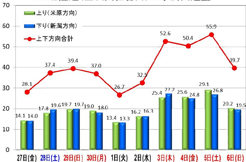
(千台/日) E8北陸道(金沢支社管内)の予測交通量
