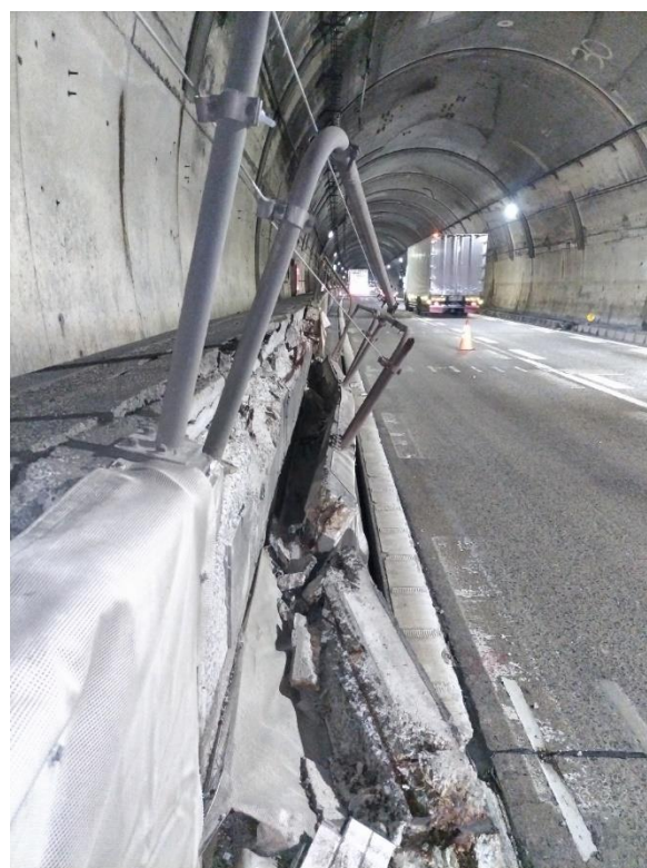
監視員通路側壁の傾倒状況(近景)
