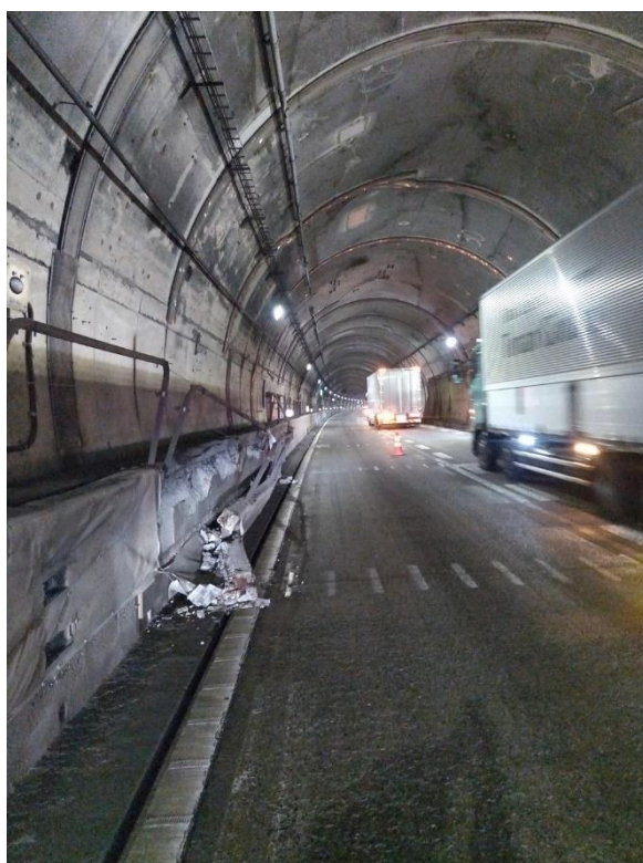
監視員通路側壁の傾倒状況(遠景)
