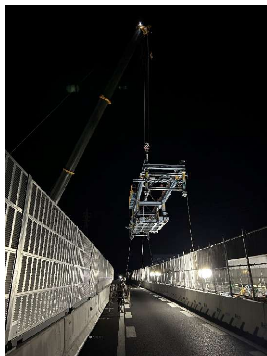
床版架設機の撤去作業状況(左:高架下から撮影、右:道路上で撮影)
