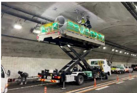
トンネル内設備点検
