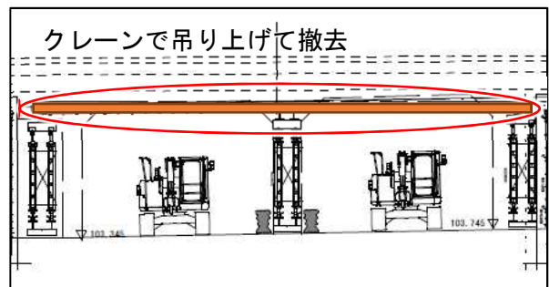
支保工のイメージ図
