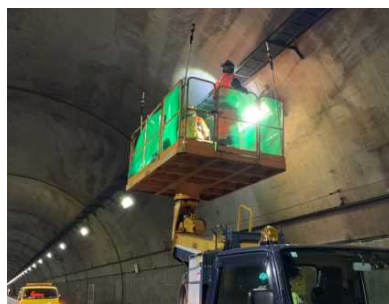
トンネル構造物点検
