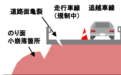
復旧イメージ 復旧前(1車線通行)
