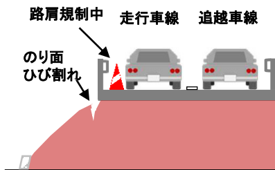
復旧イメージ 復旧前
