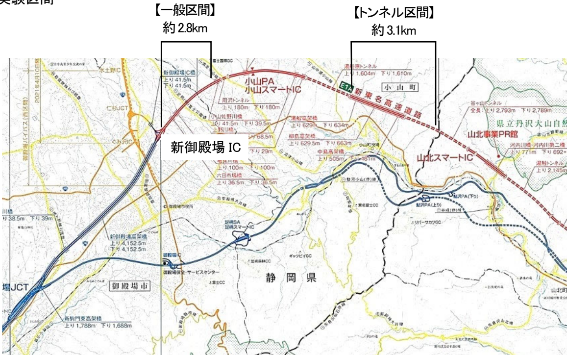
図 2 実験区間位置図
