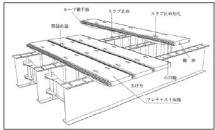
プレキャストPC床版の構造
